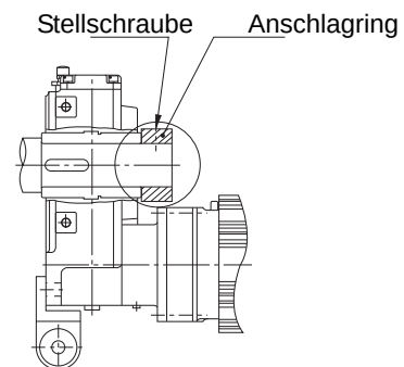
Sicherung mit Anschlagring und Stellschraube
